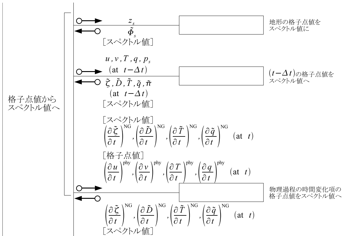
図 3.2: 力学過程 Dynamics の流れ 2. 図??の続きである. 図の見方については図??を参照せよ. ここでは格子点値をスペクトル値に変換し, それらを用いて, セミインプリシット時間積分 TimeIntegration を行っている. これ以後の処理については図??を参照されたい.
