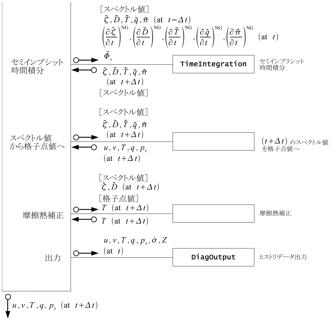
図 3.3: 力学過程 Dynamics の流れ 3. 図??の続きである. 図の見方については図??を参照せよ. ここではスペクトル値を格子点値に戻し, 摩擦熱補正をかけた後, ヒストリデータを出力し, 最後に t + \Delta t の値をサブルーチンの外に返している.
