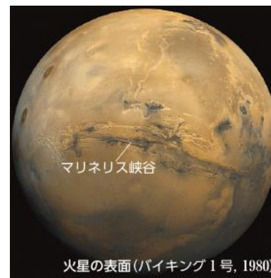
火星
